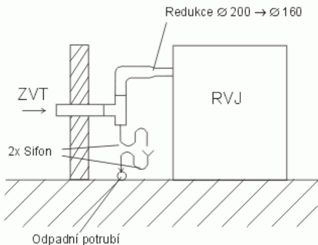
Obr. 10 - Konstrukce sifonu
