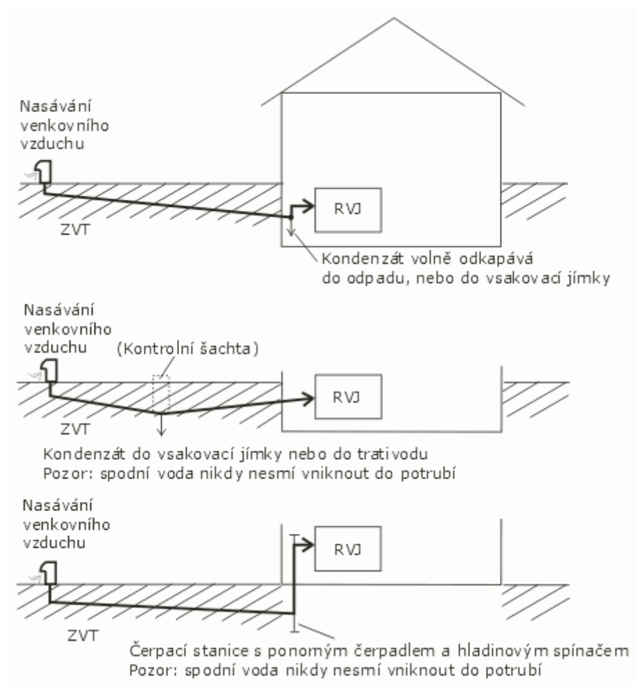
Obr. 9 - Odvádění kondenzátu
